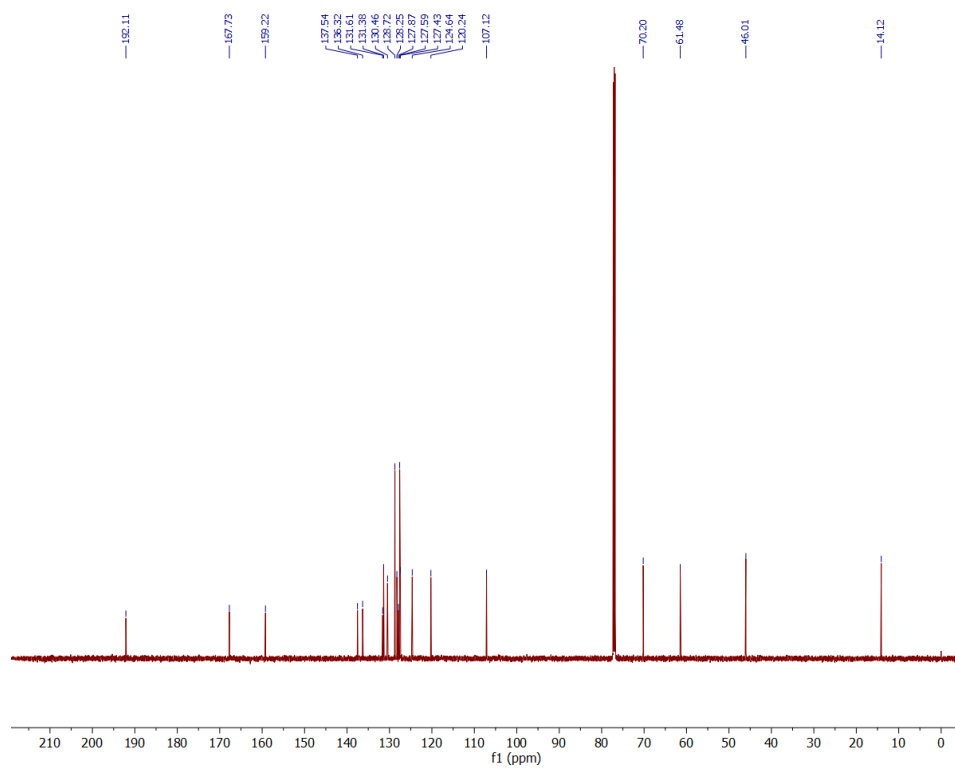
Slika D6. ^{13}\text{C} NMR spektar spoja 3 .
