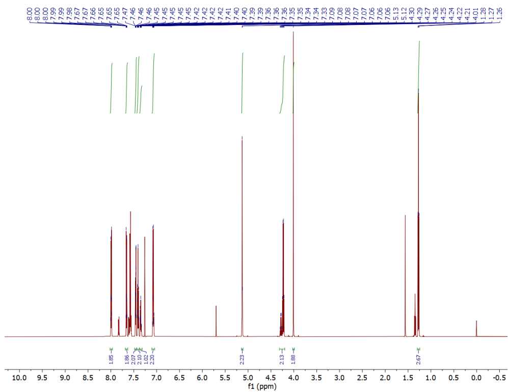
Slika D13. ^1\text{H} NMR spektar spoja 7.
