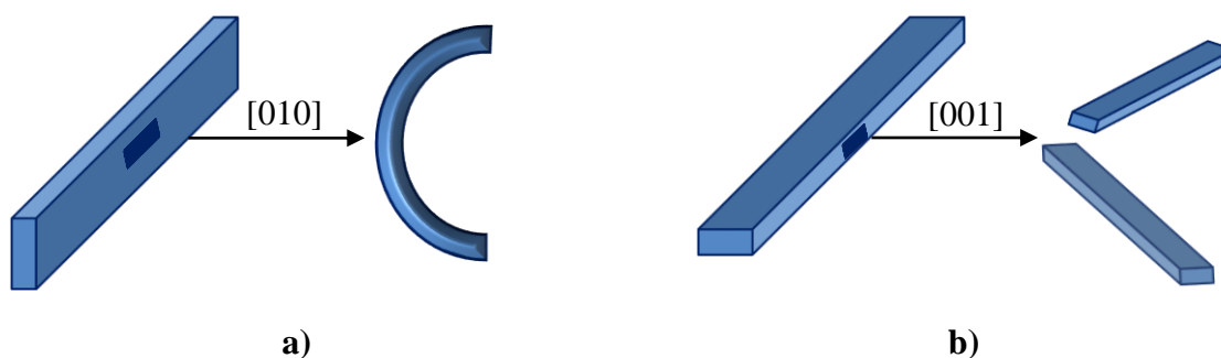
Slika 35. a) primjenom mehaničke sile okomito na plohu (010) kristal pokazuje elastičan odziv b) primjenom mehaničke sile okomito na plohu (001) dolazi do pucanja kristala
