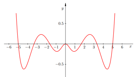
Slika 2.25: Greška interpolacijskog polinoma stupnja 6
