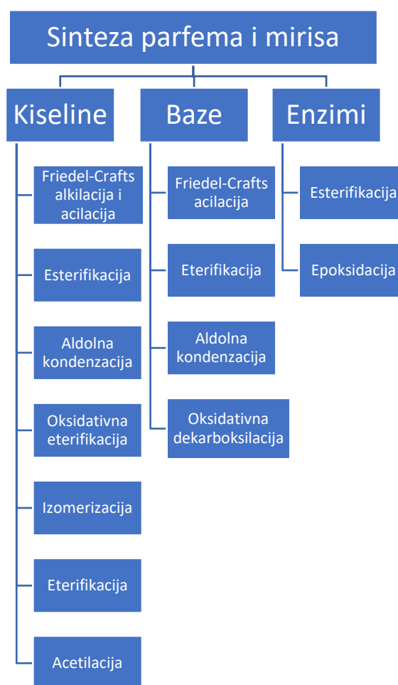
Slika 3. Reakcije transformacije
