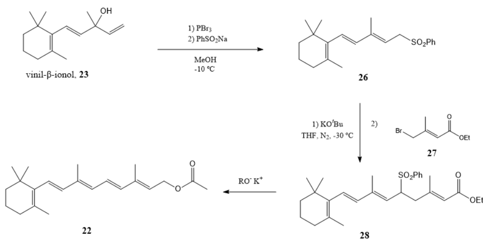
Slika 11. Shematski prikaz sinteze retinol-acetata prema Rhone-Poulenc-u 11
