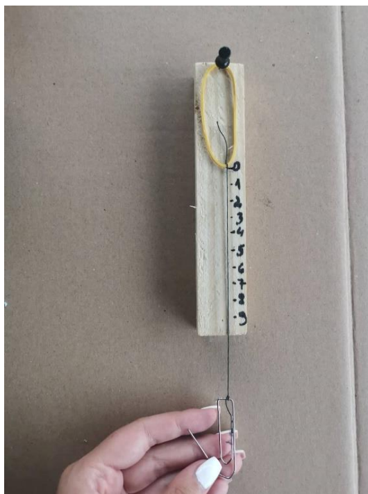
Slika 10. Dinamometar
