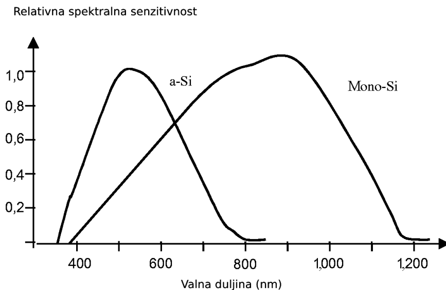
Slika 11: Relativna spektralna osjetljivost (normirana) amorfnog i monokristalne silicijske ćelije [1]
