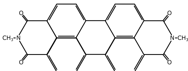
Slika 2.25: Molekula PTCDI
