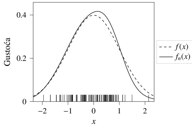
Slika 3.1: Procjena gustoće metodom jezgri za uzorak duljine n = 100 iz N(0, 1) koristeći normalnu jezgru K(x) = \frac{1}{2\pi} e^{-\frac{x^2}{2}} i h_{100} = \frac{1}{2} .
