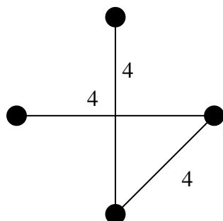
(c) T_D
