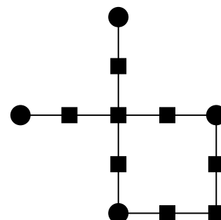
(d) M[T_D]
