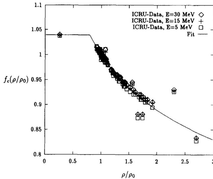
Slika 3.3. Omjer masenih sudarnih zaustavnih snaga sredstva i vode kao funkcija gustoće normirane na gustoću vode. Preuzeto od Kawrakow i sur. [27].
