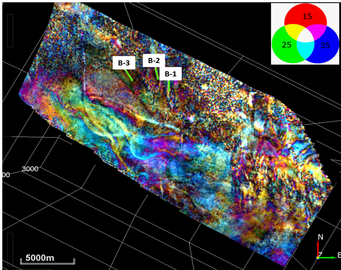
Slika 8.3.5.1.: Spektralna dekompozicija po horizontu krovine Ležišta 1 (preklapanja boja prikazana su kao najniži frekvencijski raspon u seizmičkom skupu podataka u crvenoj boji-15 Hz, dominantna frekvencija u zelenoj boji-25 Hz i najviše frekvencije u plavoj boji- 35 Hz, a predstavljaju bolju predodžbu kontinuiteta kanalnih tijela i moguću kvalitetu rezervoara).
