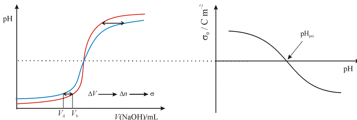
Slika 2.9. Grafički prikaz potencijometrijske kiselinobazne titracije (lijevo) na kojoj je crvenom bojom označena titracija blank otopine, a plavom titracija suspenzije te prikaz površinske gustoće naboja prikazana kao funkcije pH (desno). 27
