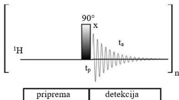
Slika 15. Pulsni slijed tehnike ^1\text{H} -NMR 34
