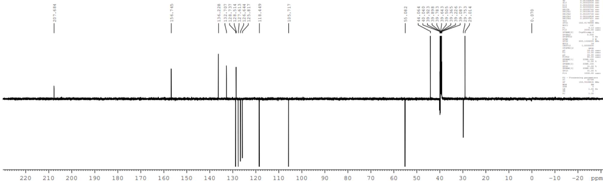
Slika D8. 13 C NMR spektar nabumetona u DMSO-d 6 na 25 °C
