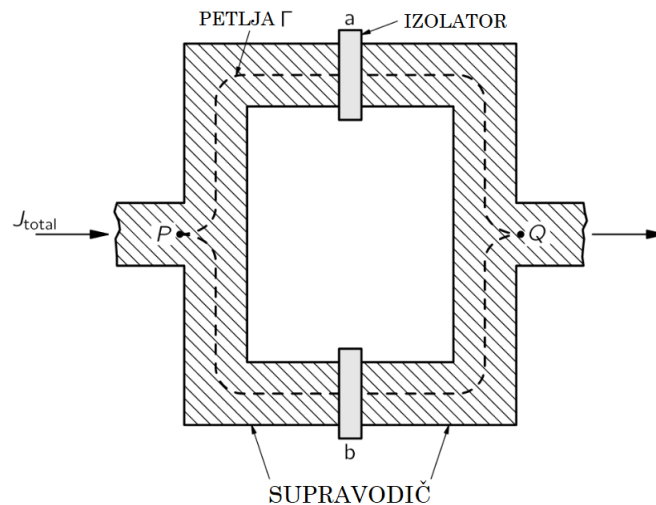
Slika 6.2. Dva Josephsonova čvora u paraleli [39]
