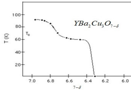
Slika 4.3: Ovisnost temperature supravodljivog prijelaza T_c o dopiranju kisikom YBa_2Cu_3O_{7-x} monokristala. [9]
