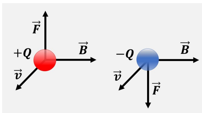
Slika 8.3: Smjerovi magnetske sile, magnetskog polja te brzine nabijene čestice za pozitivan i negativan naboj. [40]
