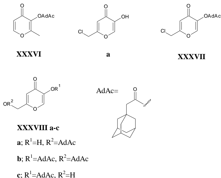
Slika 21. Strukturne formule molekula adamantilnih derivata hidropirana-4-ona s potencijalnim antitumorskim djelovanjem i klorkojske kiseline ( a ) 8
