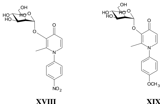
Slika 12. Strukturne formule molekula \alpha -manozidnih derivata N -aril-3,4-HP-a 74 s antiadhezijskom aktivnošću
