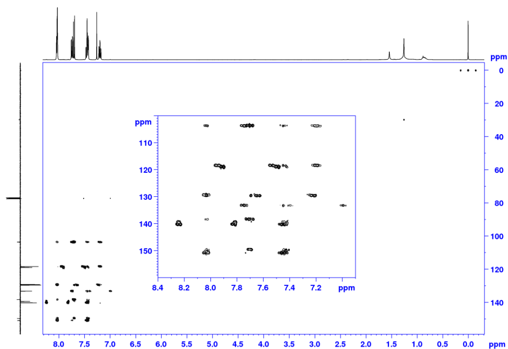
Slika D89. HMBC spektar L2I-II u \text{CDCl}_3 (400 MHz).
