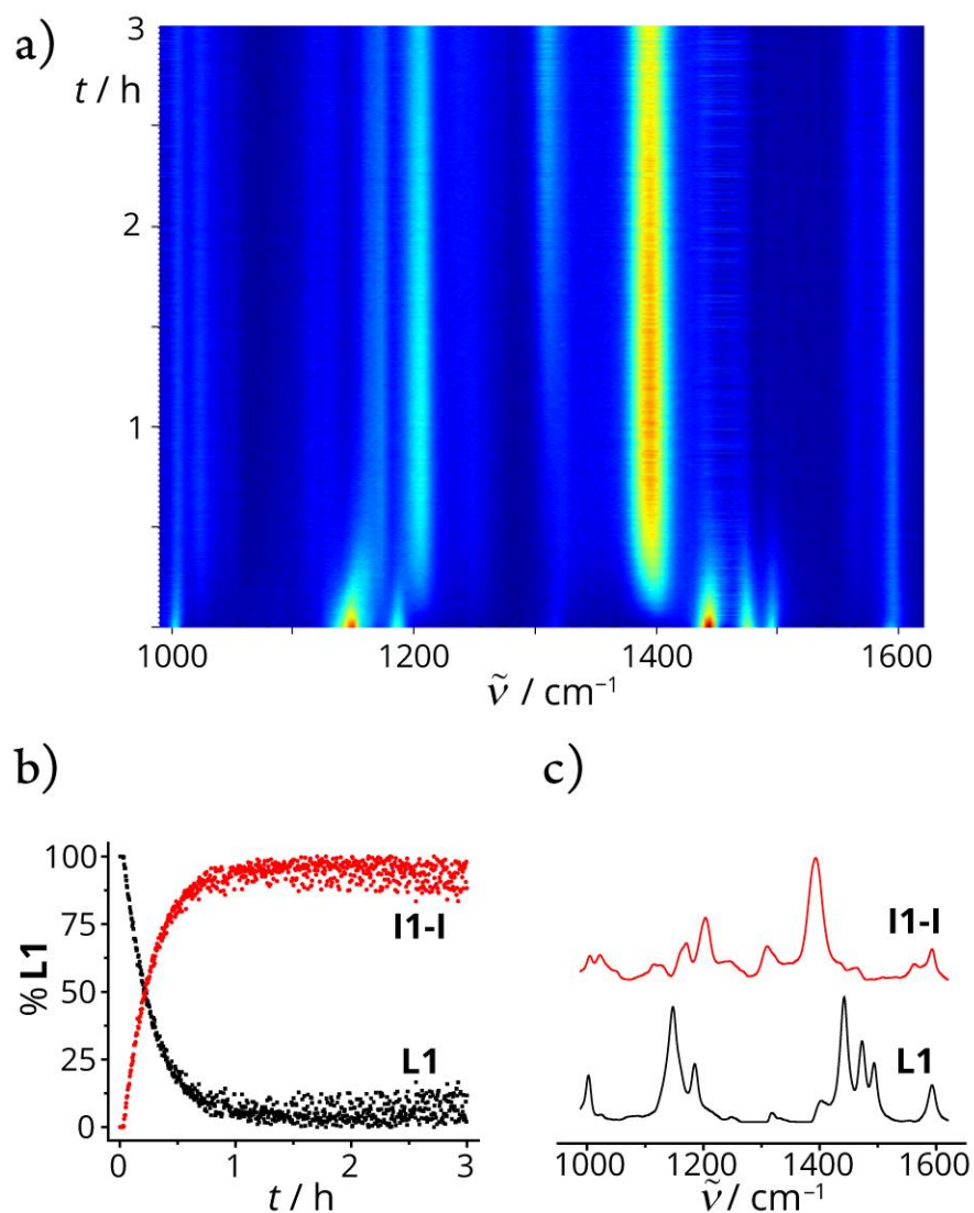
Slika D15. a) 2D prikaz vremenski razlučenog Ramanovog praćenja LAG reakcije L1 (0,4 mmol) s Pd(OAc) 2 (0,42 mmol), TsOH×H 2 O (0,42 mmol), MeCN (25 μL, 0,48 mmol) i SiO 2 (400 mg). b) Reakcijski profil dobiven MCR-ALS analizom. c) Ramanovi spektri vrsta opaženih tijekom Ramanovog praćenja reakcije dobiveni MCR-ALS analizom.
