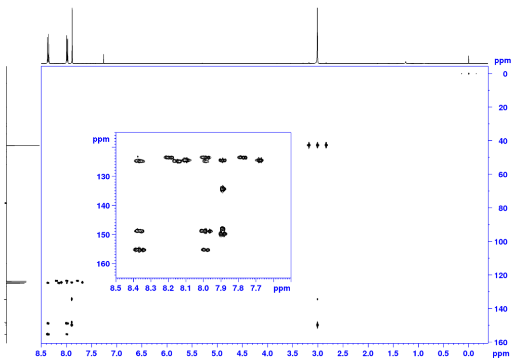
Slika D151. HMBC spektar L8Cl-IV u \text{CDCl}_3 (400 MHz).
