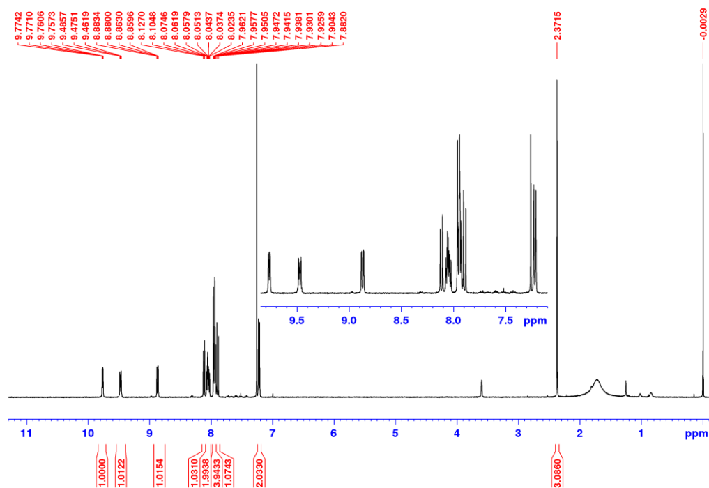
Slika D181. ^1\text{H} NMR spektar sirove reakcijske smjese NG reakcije L9 (0,5 mmol) i \text{TsOH}\times\text{H}_2\text{O} (0,5 mmol) u \text{CDCl}_3 (400 MHz).
