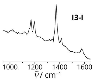
Slika D32. Ramanov spektar 13-I u čvrstom stanju.
