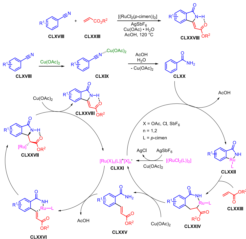
Shema 28. Priprava Z-3-metilenizindolina katalizirana rutenijevim kompleksom [(RuCl_2(p\text{-cimen}))_2]
