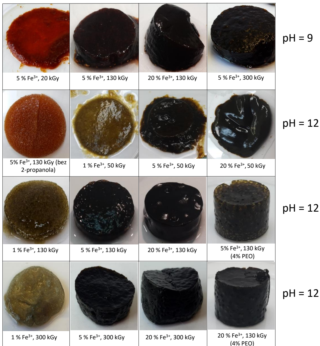
Slika 55. Fotografije odabranih kompozitnih PEO/Fe-oksida hidrogelova dobivenih iz suspenzija s različitim početnim koncentracijama Fe 3+ pri različitim dozama; sve prekursorske suspenzije su pripremljene iz 1,85 %-tnih PEO (400 000) otopina i uz dodatak 0,2 mol dm -3 2-propanola (osim ako nije drugačije naznačeno) pri pH = 9 ili 12
