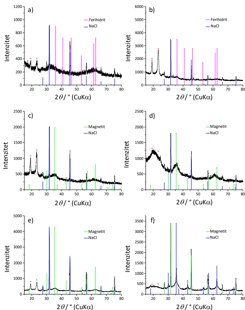
Slika 57. XRD analiza neozračenog prekursora PEO400-0/12/5/1,85/0,2 (a) i PEO/Fe-oksida gelova pri pH \sim 12: b) PEO400-50/12/5/1,85/0,2, c) PEO400-130/12/5/1,85/0,2, d) PEO400-300/12/5/1,85/0,2, e) PEO400-130/12/20/1,85/0,2, f) PEO400-300/12/20/1,85/0,2; crvenim točkama označene su linije čistog praha PEO (ICDD kartice korištene za kvalitativnu analizu: Fe 3 O 4 19-0629, ferihidrit 29-0712, NaCl 5-0628)
