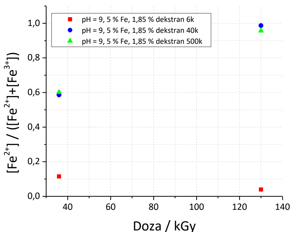
Slika 51. Ovisnost stupnja redukcije Fe 3+ određen kompleksiranjem s 1,10-fenantrolinom u \gamma -ozračenim suspenzijama uz dekstrane različitih molekulskih masa s 5 % Fe 3+ , pri pH = 9 i uz 0,2 mol dm -3 2-propanola kao funkcija apsorbirane doze
