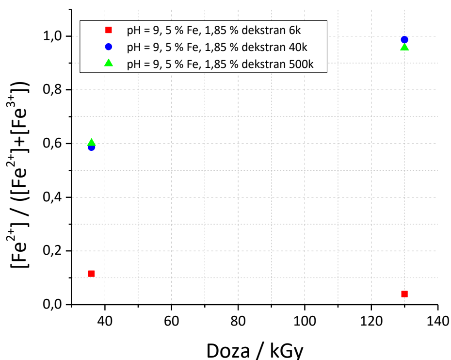
Slika 51. Ovisnost stupnja redukcije \text{Fe}^{3+} određen kompleksiranjem s 1,10-fenantrolinom u \gamma -ozračenim suspenzijama uz dekstrane različitih molekulskih masa s 5 % \text{Fe}^{3+} , pri pH = 9 i uz 0,2 \text{ mol dm}^{-3} 2-propanola kao funkcija apsorbirane doze
