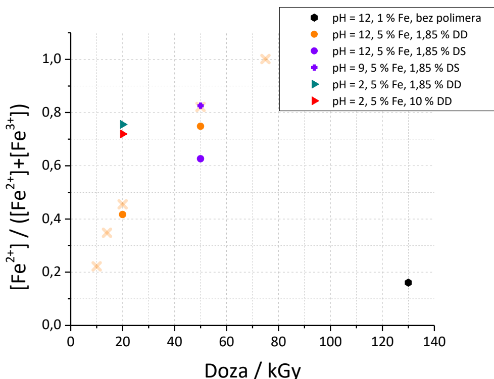
Slika 50. Ovisnost stupnja redukcije \text{Fe}^{3+} određen kompleksiranjem s 1,10-fenantrolinom u \gamma -ozračenim suspenzijama različitih pH uz DEAE-dekstran i dekstran sulfat kao funkcija apsorbirane doze; narančastim, transparentnim križićima označeni su rezultati određivanja željeza prethodno dani na slici 32 (5 % \text{Fe}^{3+} , 1,85 % DEAE-dekstran, 0,2 \text{ mol dm}^{-3} 2-propanol, \text{pH} = 9 ) radi lakše usporedbe
