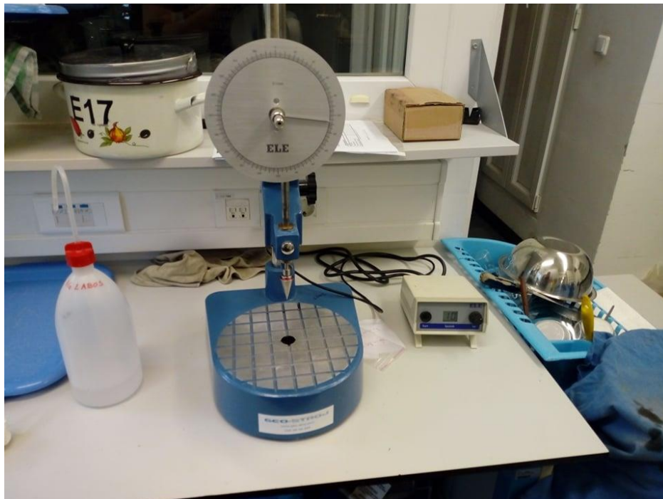
Slika 3.14. Konusni penetrometar.
