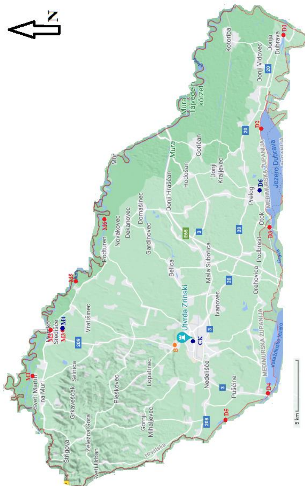
Slika 5: Karta Međimurja s točkama uzorkovanja; crvene – uzorci iz rijeka, plave – uzorci iz gradskih vodovoda, narančasta – uzorak bunarske vode
