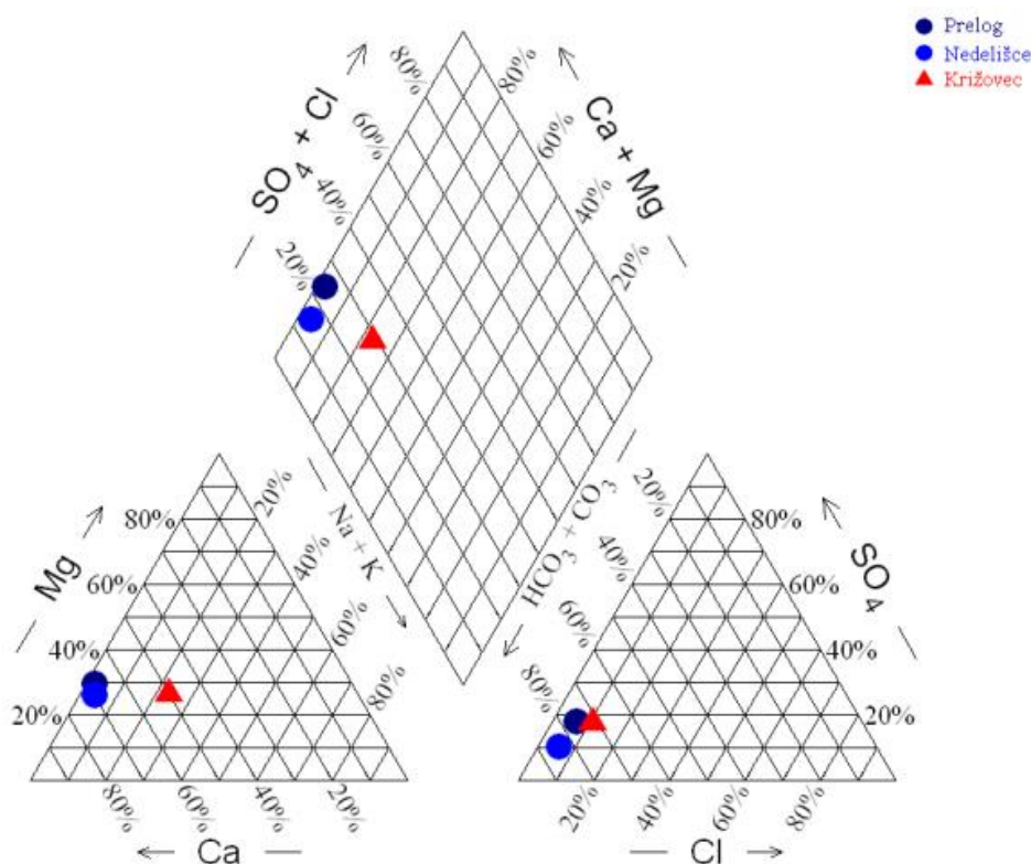
Slika 2: Piperov dijagram voda u vodnom tijelu Međimurje [9]
