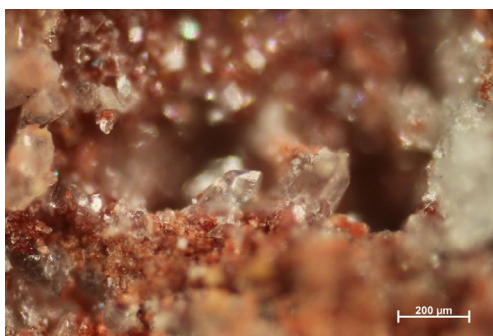
Slika 19. Kristal kremenca u šupljini uzorka promatran pod lupom
