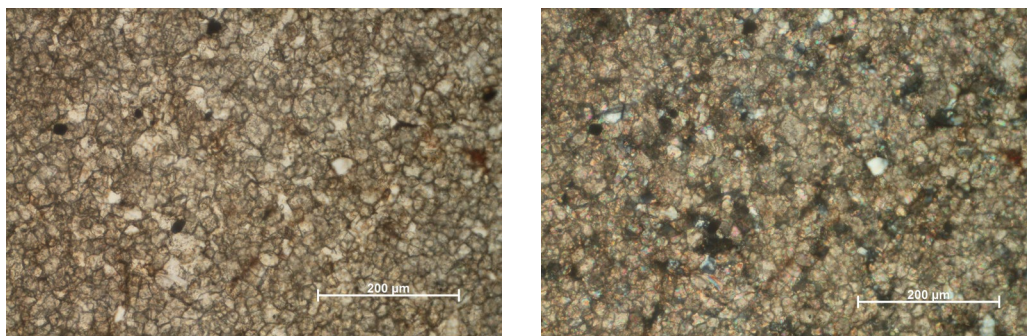
Slika 24. Fotomikrografija Preparata 4 bez analizatora i s analizatorom; dolomitna stijena
