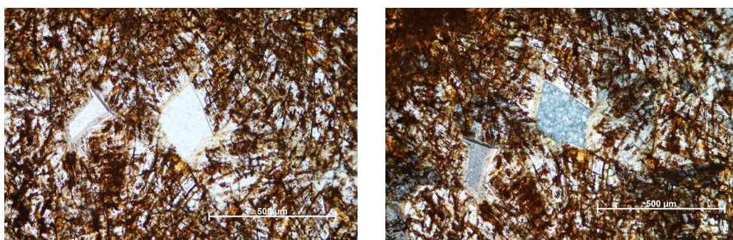
Slika 25. Fotomikrografija Preparata 5 bez analizatora i s analizatorom; agregati kalcita i goethita
