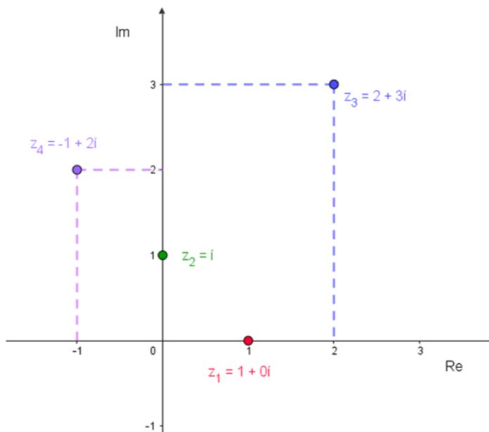
Slika 2.2: Prikaz broja z = x + yi u Gaussovoj ravnini
