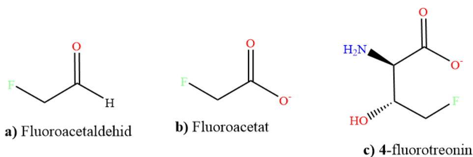
Slika 9. Strukture sekundarnih metabolita bakterije S. cattleya ; toksičnog fluoroacetata (b) i jedine prirodne aminokiseline koja sadrži fluor, 4-florotreonina (c) čiji je zajednički prekursor fluoroacetaldehyd (a). Slika napravljena pomoću ChemDraw softvera.
