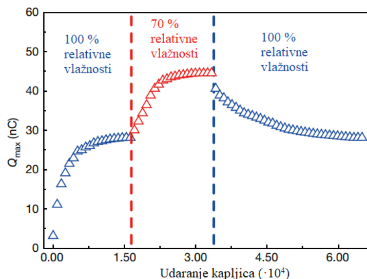
Slika 15: Grafički prikaz ovisnosti vrijednosti površinskih naboja o broju kapljica koje udare u uređaj za različite vrijednosti relativne vlažnosti [24].
