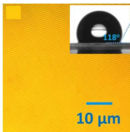
Slika 16: Utisnuti PDMS sloj uslikan optičkim mikroskopom. Boja je dobivena interferencijom svjetlosti zbog uzorka sloja. Umanjena slika pokazuje kontaktni kut kapljice vode sa slojem (~118°) [33].
