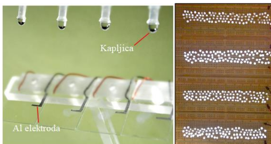
Slika 14: Slika postava četiri DEG-a na koje padaju kapljice vode (lijevo). Sto svjetlosnih dioda zasvijetli kada jedna kapljica padne na DEG (desno) [24].
