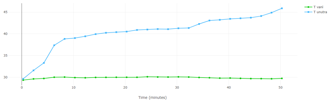
Slika 5.3.3 Odnos temperatura unutar i izvan plasteinika za vrijeme mjerenja.
