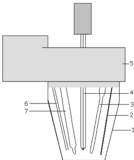
Slika 3.4. Shema troelektrodnog sustava: 1 - elektrochemijska ćelija, 2 - protuelektroda, 3 - referentna elektroda, 4 - staklena kapilara, 5 - poklopac, 6 - cjevčica za uvođenje dušika, 7 - rotirajuće teflonsko miješalo.
