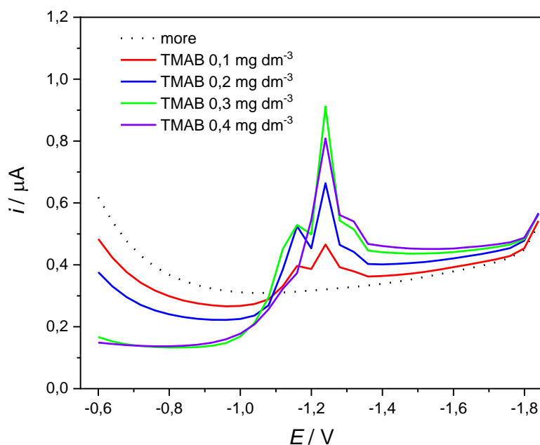
Slika 4.11. AC voltamogrami različitih koncentracija TMAB. E_a = -0,6 \text{ V} , t_a = 60 \text{ s} .
