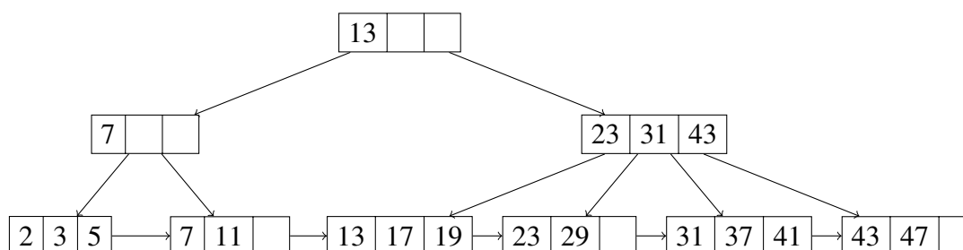
Slika 4.6: B-stablo
