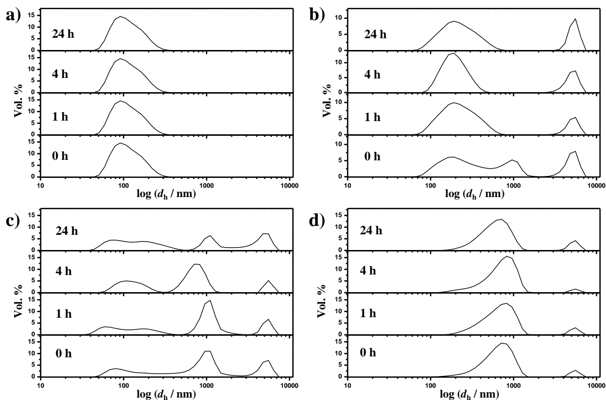
Slika 47. Repräsentativne raspodjele veličine a) TiO 2 nanočestica, b) TiO 2 nanopločica, c) titanatnih nanocjevčica i d) titanatnih nanožica koncentracije 200 mg L -1 suspendiranih u otopini 8 mmol dm -3 Na 2 HPO 4 i 100 mg L -1 albumina iz goveđeg seruma nakon 0, 1, 4 i 24 h pri pH 7,4 i 25 °C.
