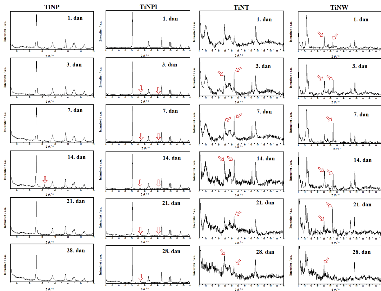
Slika 55. Difraktogrami praha TiO 2 nanočestica (TiNP), TiO 2 nanopločica (TiNPI), titanatnih nanocjevčica (TiNT) i titanatnih nanožica (TiNW) nakon 1, 3, 7, 14, 21 i 28 dana inkubacije u SBF-u koji sadrži 5 g L -1 albumina iz goveđeg seruma (BSA) pri 25 °C. Crvene strelice označuju difrakcijske maksimume koji pripadaju kalcijevim fosfatima.
