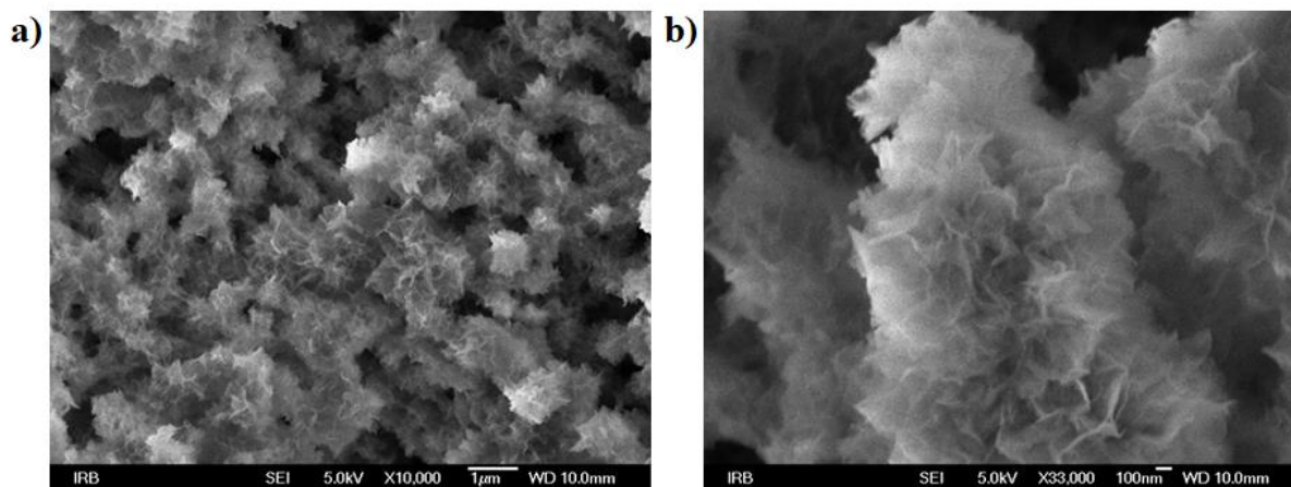
Slika 64. SEM mikrofografije pri a) manjem i b) većem povećanju taloga nastalog nakon 60 min u kontrolnom sustavu: c(\text{CaCl}_2) = c(\text{Na}_2\text{HPO}_4) = 4 \cdot 10^{-3} \text{ mol dm}^{-3} pri 25 \text{ }^\circ\text{C} i \text{pH}_{\text{poč}} = 7,4 .
