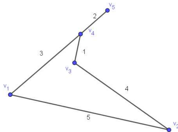
Slika 2.4: Težinski graf
