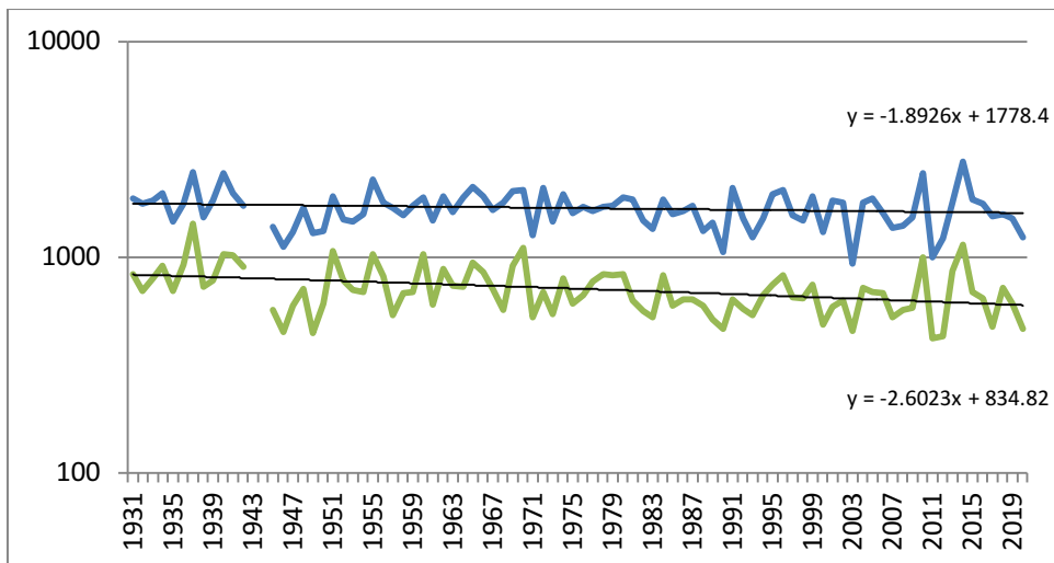
Sl. 6. Godišnji srednji minimumi i maksimumi protoka na stanicama Stara Gradiška, Slavonski Brod i Županja stepenica 1931. – 2020. godine
