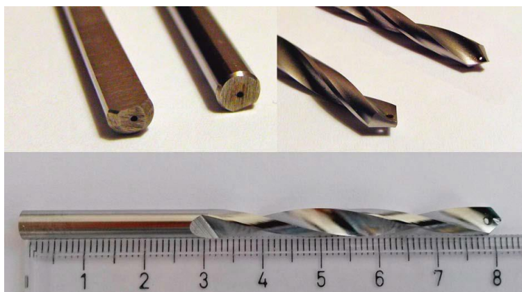
Slika 26. Primjer medicinskoga svrdla s unutarnjim hlađenjem
