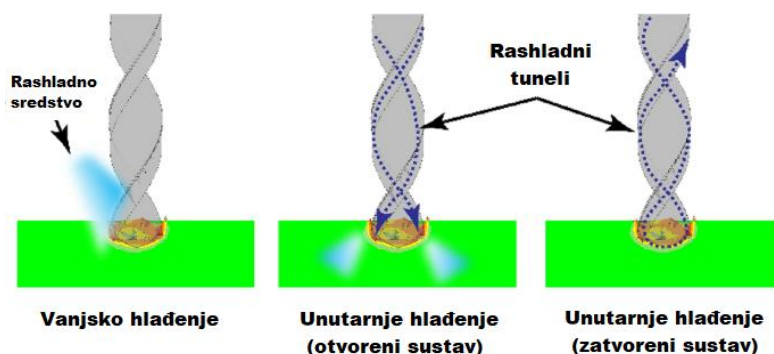
Slika 24. Sustavi za hlađenje pri bušenju medicinskim svrdlom
