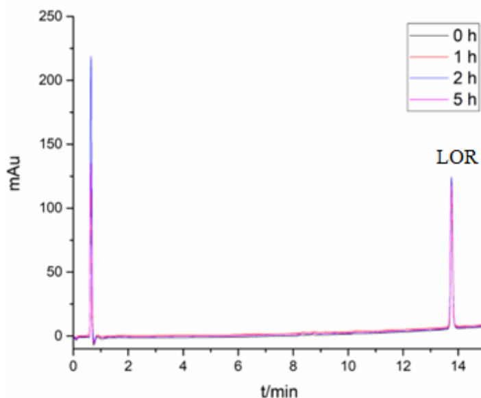
Slika 13. Kromatogram LOR nakon razgradnje u kiselim uvjetima u vremenskim intervalima od 0 h, 1 h, 2 h i 5 h uz zagrijavanje na 80^\circ\text{C} , pri valnoj duljini od 275 nm
