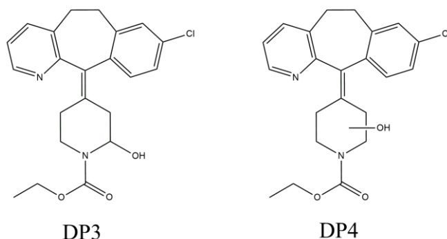
Slika 28. Predložene strukture degradanata DP3 i DP4 dobivenih nakon razgradnje LOR u oksidativnim uvjetima
