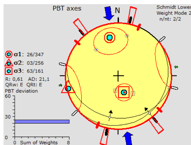
Slika 5-12. Stereogram proračuna vektora glavnih osi napreznja za reversne rasjede na području istraživanja (pomoću programa Win_Tensor ).
