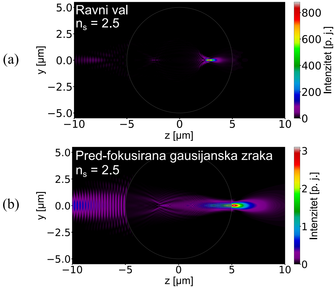
Slika 6.22: Prikaz intenziteta električnog polja u y-z ravnini pri raspršenju svjetlosti ( \lambda = 515 nm) na mikrosferi visokog indeksa loma n_s = 2.5 i polumjera R = 5 \mu\text{m} . Smjer propagacije je u pozitivnom smjeru z -osi. (a) Upadna svjetlost je ravni val. Nastali fotonski nanomlaz duboko je unutar mikrosfere. (b) Upadna svjetlost je gausijanska zraka čiji je polumjer pojasa w_0 = 0.7 \mu\text{m} , a pozicija pojasa z_0 = -13 \mu\text{m} (pred-fokusiranje). Nastali fotonski nanomlaz nalazi se izvan mikrosfere.
