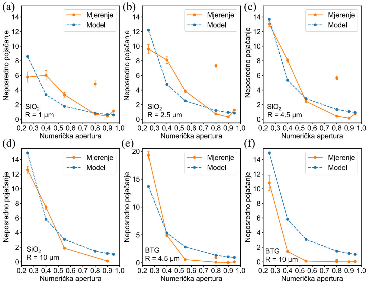
Slika 6.39: Ovisnost neposrednog pojačanja o NA mikroskopskog objektiva za različite polumjere SiO 2 i BTG mikrosfera, u usporedbi s modelom efektivne numeričke aperture (NA eff ). Korišteno je koleksijsko vlakno promjera 100 μm.
