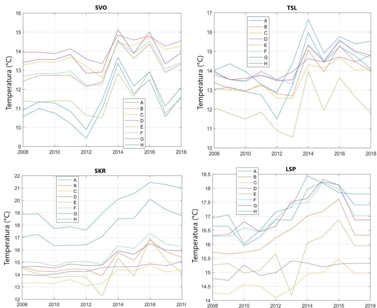
Slika 4.3.2. Sezonske srednje vrijednosti modelirane pridnene temperature mora po ribolovnim zonama (SVO: siječanj - veljača - ožujak; TSL: travanj - svibanj - lipanj; SKR: srpanj - kolovoz - rujanj; LSP - listopad - studeni - prosinac)
