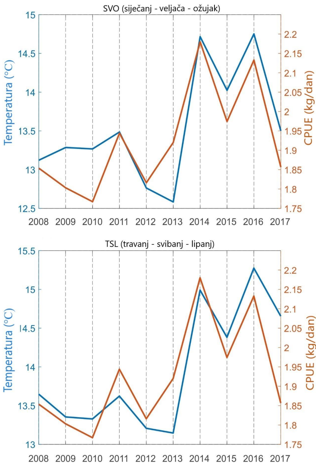
Slika 4.4.7. Vremenski niz zimske (SVO) i proljetne (TSL) pridnene temperature mora i CPUE (kg/dan) hlapa za grupirane ribolovne zone srednjeg Jadrana (zone C, G i F)
