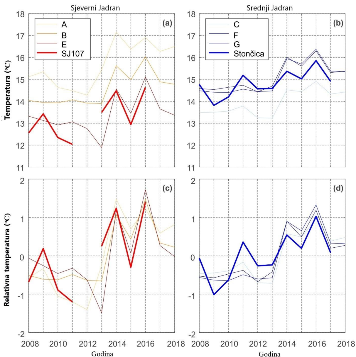
Slika 4.2.1. Usporedba modela i mjerenja srednje godišnje vrijednosti temperature mora na: (a) mornoj postaji SJ107 i ribolovnim zonama sjevernog Jadrana (ribolovne zone A, B i E); (b) mjerna postaja Stončica i srednje Jadranske ribolovne zone (ribolovne zone C, F, G). (c)-(d) isto kao (a)-(b), ali s uklonjenim srednjim vrijednostima.
