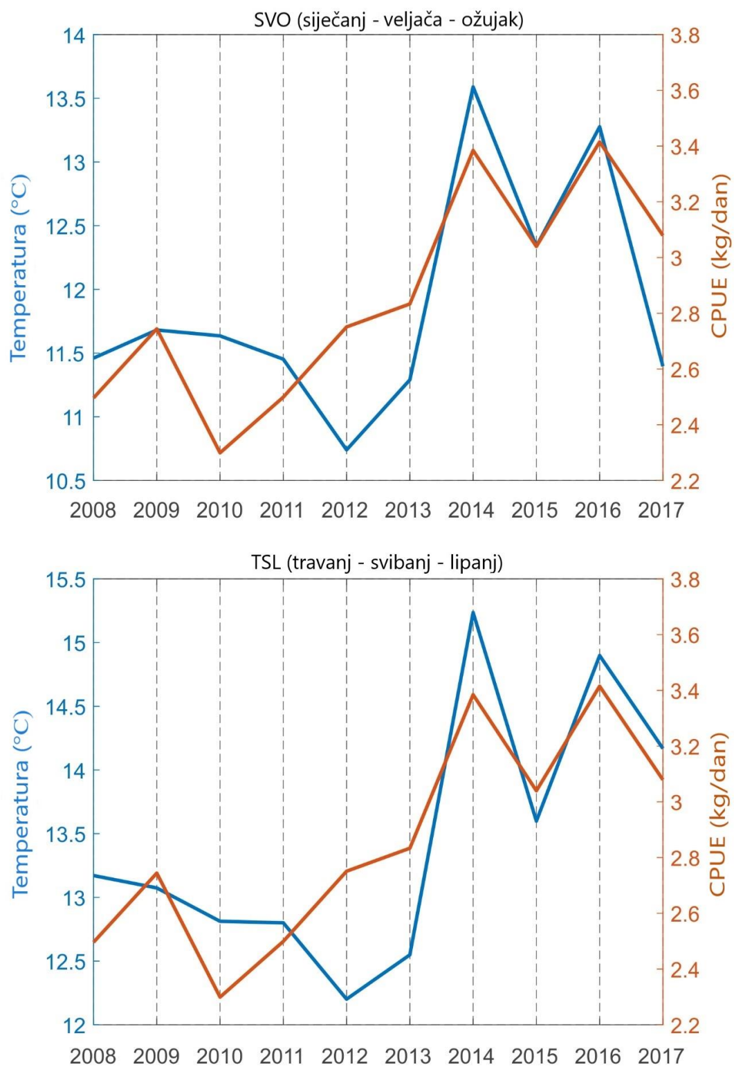
Slika 4.4.6. Vremenski niz zimske (SVO) i proljetne (TSL) pridnene temperature mora i CPUE (kg/dan) hlapa za grupirane ribolovne zone sjevernog Jadrana (zone A, B i E)
