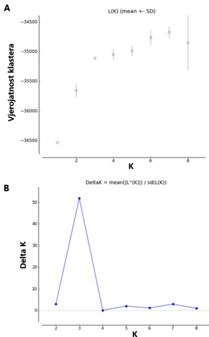
Slika 4.8.2. Prikaz broja klastera za set podataka o populaciji hlapa Homarus gammarus . (A) Srednja vrijednost \pm standardna devijacija vjerojatnosti svakog klastera (K); (B) vrijednosti Delta K izračunate kao srednja vrijednost stope promjene drugog reda vjerojatnosti K podijeljena sa standardnom devijacijom vjerojatnosti K. K s najvećom vrijednosti Delta K predstavlja najvjerojatniji broj populacija.
