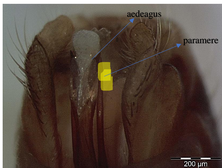
Slika 93. Allogamus auricollis braueri . Genitalni aparat mužjaka, ventralna strana, izvor rijeke Une, 15.10.2014. (leg. A. Čukušić, A. Delić) zbirka „Trichoptera NiP“, označeno – aedeagus i paramere (foto M. Kučinić).
