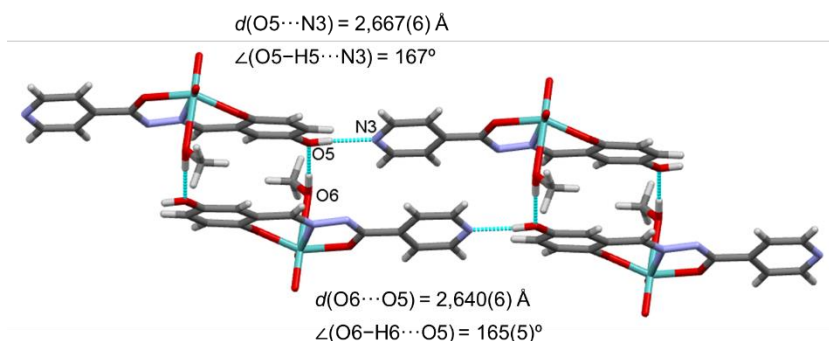
Slika 107. Prikaz vodikovih veza u spoju [\text{MoO}_2(5\text{OHSIH})(\text{MeOH})] .
