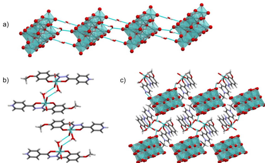
Slika 86. a) Povezivanje oktamolibdatnih jedinica preko kristalizacijske vode u 1D lance b) dimer kompleksnog kationa c) prikaz pakiranja duž osi a u spoju [\text{MoO}_2(\text{H}_24\text{OMeSIH})(\text{H}_2\text{O})]_2[\text{Mo}_8\text{O}_{26}] \cdot 2\text{MeCN} \cdot 3\text{H}_2\text{O} (na zasebnim slikama izostavljene su kristalizacijske vode radi jednostavnijeg prikaza).
