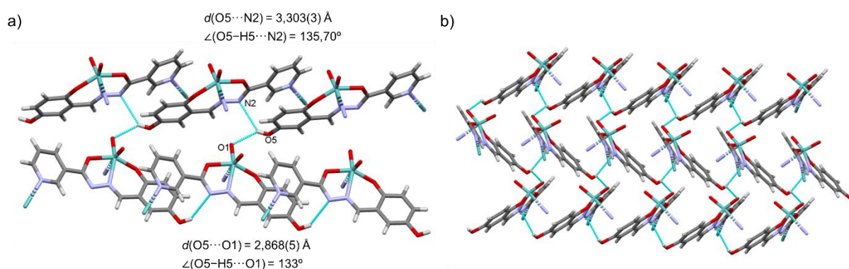
Slika 105. Prikaz vodikovih veza u: a) [\text{MoO}_2(\text{5OHSalNH})]_n i b) slaganje u supramolekulska 3D mrežu.
