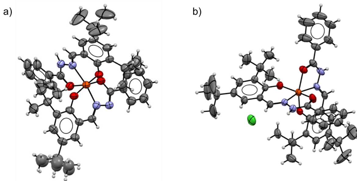
Slika 12. Struktura kompleksa: a) [\text{Fe}(\text{HL})(\text{L})] \cdot \text{EtOH} \cdot \text{H}_2\text{O} i b) [\text{Fe}(\text{HL})_2]\text{Cl} \cdot 1,5\text{MeOH} \cdot 0,5\text{EtOH} pri čemu su radi jednostavnosti prikaza uklonjene molekule otapala.
