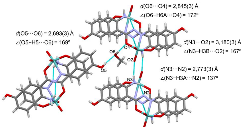
Slika 108. Prikaz vodikovih veza u spoju [\text{MoO}_2(5\text{OMeSal-2HBNH}_2)]_2 \cdot 2\text{MeOH} .
