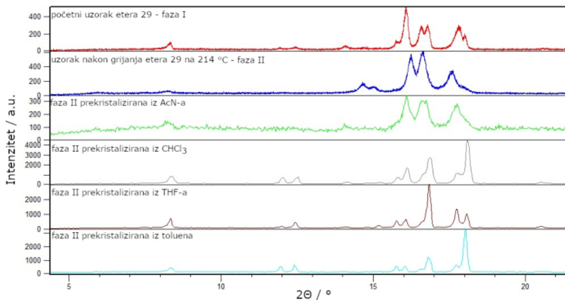
Slika 64. Usporedba difraktograma etera 29 (crvena linija), uzorka nastalog nakon zagrijavanja spoja 29 do 214 °C (plava linija) te uzoraka nastalih nakon prekrizalizacije zagrijanog uzorka u acetonitrilu (zelena linija), kloroformu (siva linija), tetrahidrofuranu (smeđa linija) te toluenu (svijetlo plava linija).
