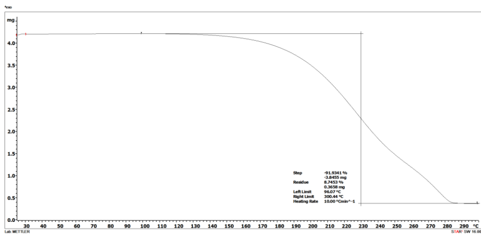
Slika D55. Termogram (nba4Ian)(135tfib).
