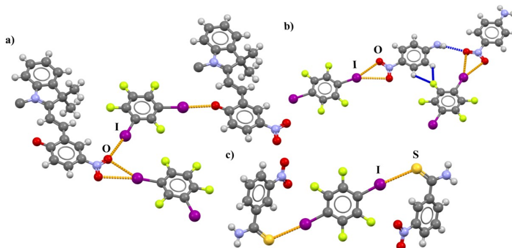
Slika 18. Prikaz povezivanja odabranih višekomponentnih sustava s perhalogeniranim donorima halogenske veze: a) PUDBAU 87 s istaknutim halogenskim vezama O \cdots I, b) JEJBM 3 , s istaknutim halogenskim vezama O \cdots I (narančasto) i vodikovim vezama (plavo), c) KUWQUQ 88 , s istaknutim halogenskim vezama S \cdots I.
