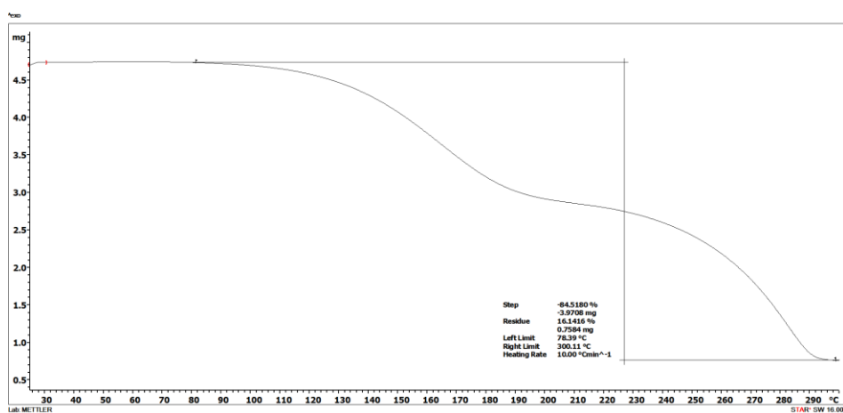
Slika D54. Termogram (nba4Ian)(13tffb).
