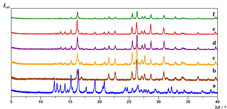
Slika D21. Usporedba difraktograma: a) nba4Clan , b) 14tfib , c) produkt dobiven mljevenjem nba4Clan i 14tfib u stehiometrijskom omjeru 1:1 uz dodatak MeCN ( d = 5 mm, t = 30 min, m_{total} = 100 mg), d) produkt dobiven mljevenjem nba4Clan i 14tfib u stehiometrijskom omjeru 1:1 uz dodatak MeCN ( d = 5 mm, t = 60 min, m_{total} = 100 mg), e) produkt dobiven mljevenjem nba4Clan i 14tfib u stehiometrijskom omjeru 1:1 uz dodatak MeNO 2 ( d = 7 mm, t = 30 min, m_{total} = 100 mg), f) produkt dobiven mljevenjem nba4Clan i 14tfib u stehiometrijskom omjeru 1:1 uz dodatak MeNO 2 ( d = 7 mm, t = 60 min, m_{total} = 100 mg).
