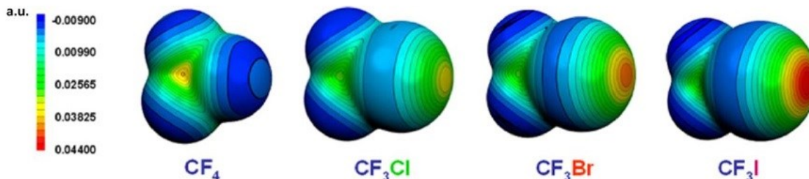
Slika 2. Elektrostatski potencijal u Hartree-ima mapiran na izoplohu elektronske gustoće ( \rho_{el} = 0,001 elektron Bohr -3 ) u molekulama perfluoriranih halogenalkana (CF 4 , CF 3 Cl, CF 3 Br, CF 3 I) 17
