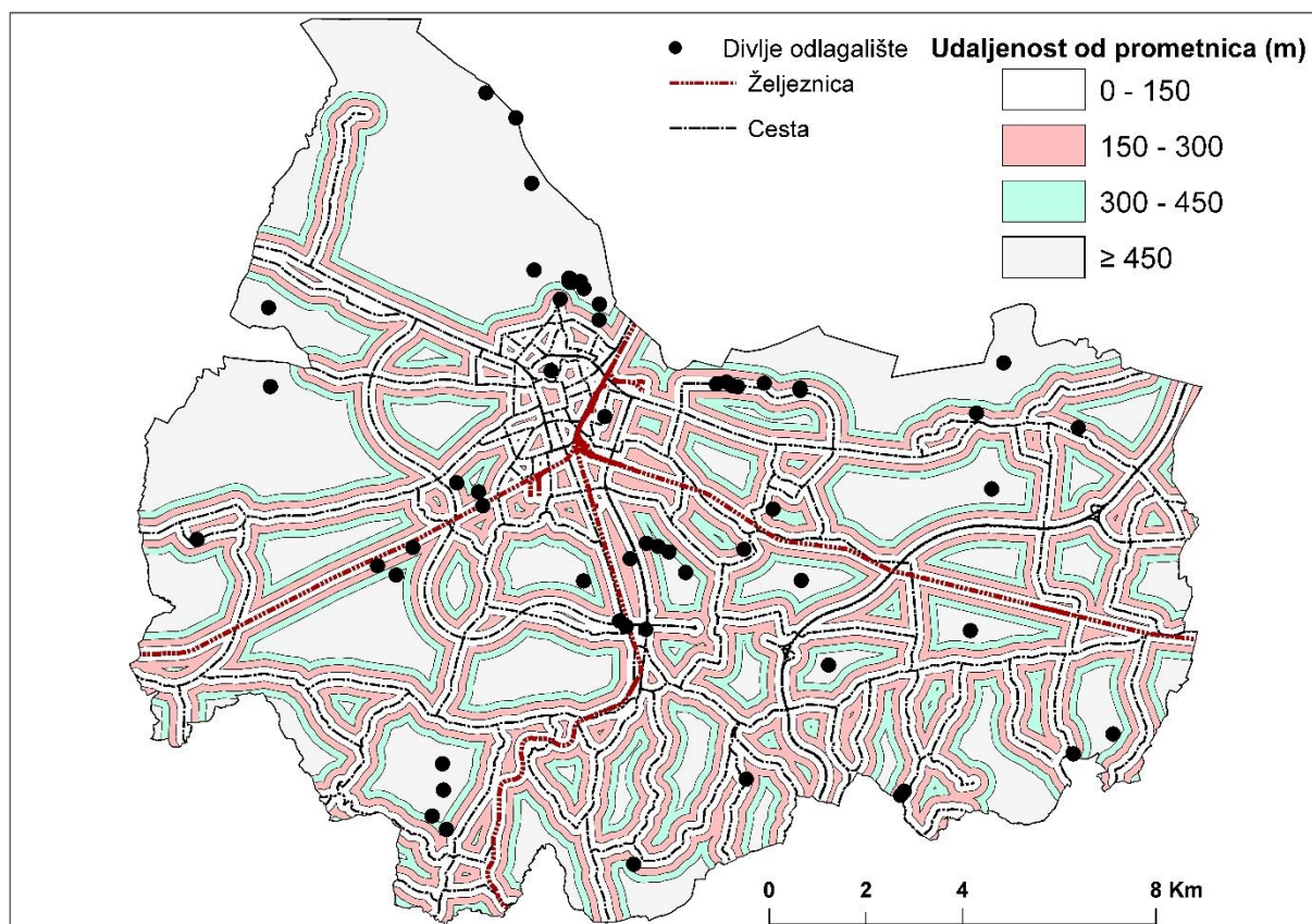
Sl.11. Pojava divljih odlagališta s obzirom na udaljenost od važnijih prometnica
