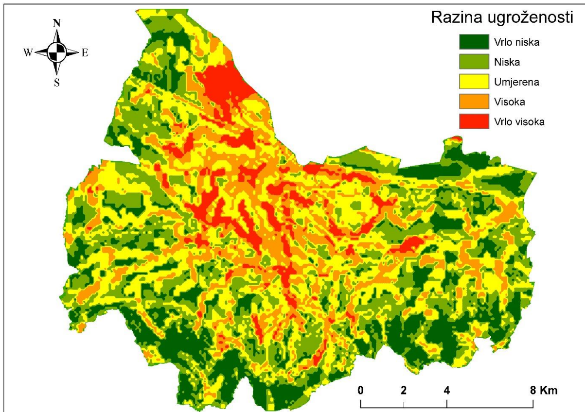
Sl.18. Kartografski prikaz ugroženosti šireg varaždinskog područja divljim odlagalištima Izvor: izradio autor prema podacima iz vlastite arhive
