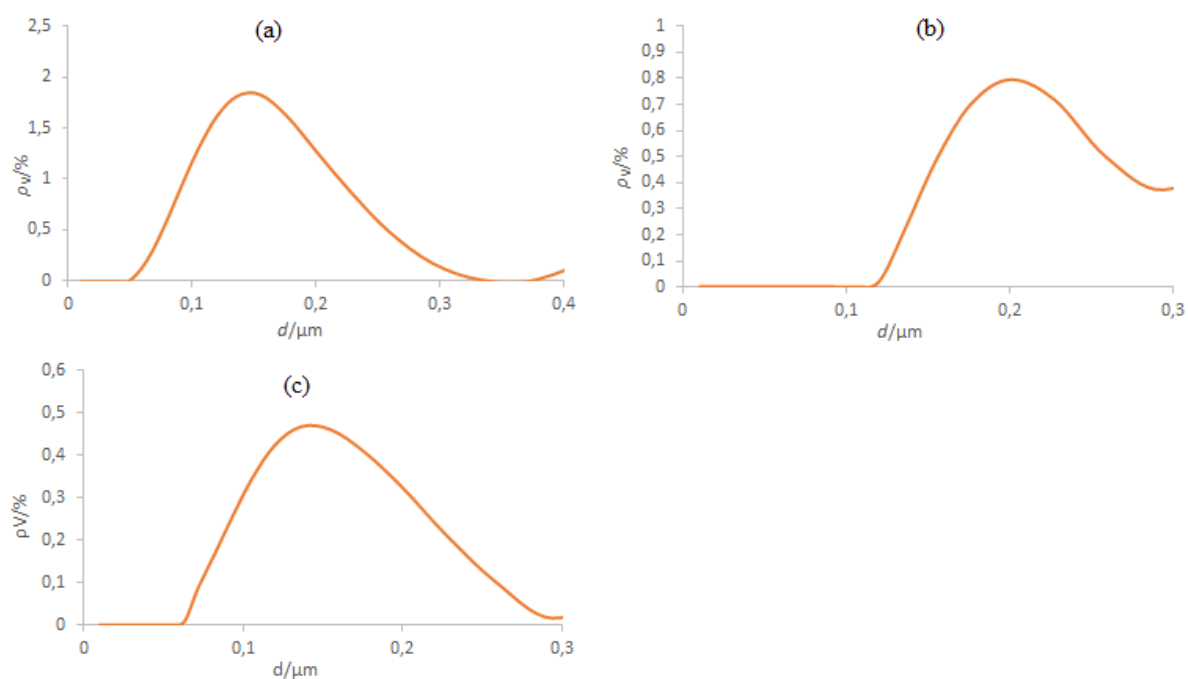
Slika 43. Raspodjela veličine čestica \text{TiO}_2 po volumenu za \text{pH} = 3 i I_c = 0,001 \text{ mol dm}^{-3} , (a) T-250, (b) T-50-70 i (c) T-15
