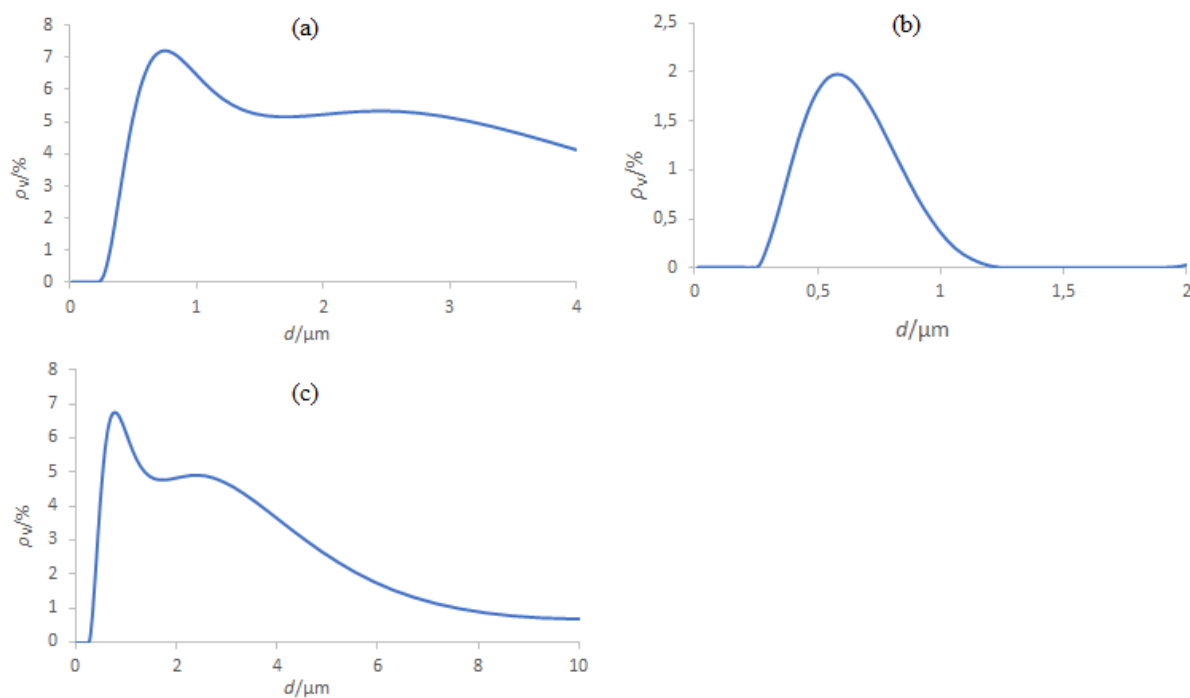
Slika 42. Raspodjela veličine čestica \text{SiO}_2 po volumenu za \text{pH} = 7 i I_c = 0,001 \text{ mol dm}^{-3} , (a) S-1000, (b) S-200 i (c) S-80
