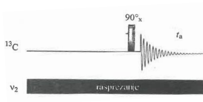
Slika 2.2.7. Pulsni slijed tehnike „off-resonance“ ^{13}\text{C} NMR. 50
