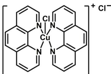
Slika 9. Molekulska struktura akceptora halogenske veze \text{CuCl}(\text{phen})_2\text{Cl}
