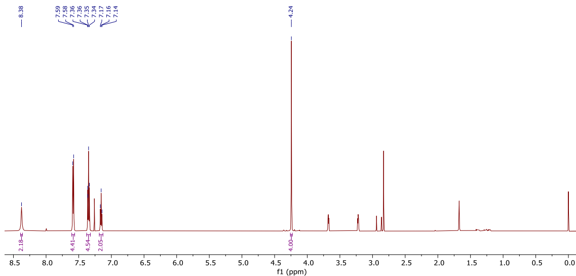
Slika D16. ^1\text{H} NMR spektar L5, \text{CDCl}_3 , 600 MHz, 25 °C.
