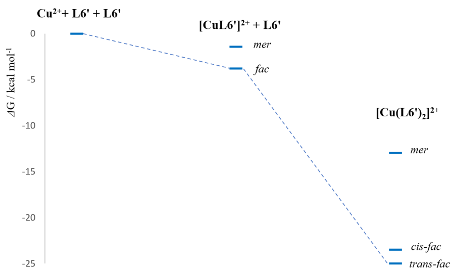
Slika 42. Dijagram promjene slobodne Gibbsove energije prilikom vezanja liganda L6' na ion bakra(II). (SMD)/M05-2X/6-31+G(d)/LanL2DZ + ECP metoda, acetonitril, 25 °C.
