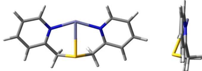
Slika 51. Razlike u mer vezanju metalnog iona između kisika i sumpora. Pogled na ML strukture iz dva smjera. (SMD)/M05-2X/6-31+G(d)/LanL2DZ + ECP metoda, acetonitril, 25 °C.
