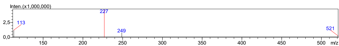
Slika D34. ESI-MS spektri L3. Pozitivan sken (gore) i negativan sken (dolje), metanol.
