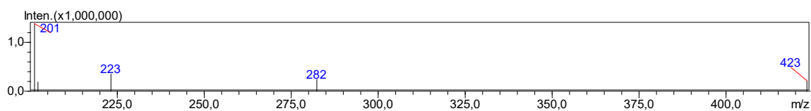
Slika D32. ESI-MS spektri L1. Pozitivan sken (gore) i negativan sken (dolje), metanol.
