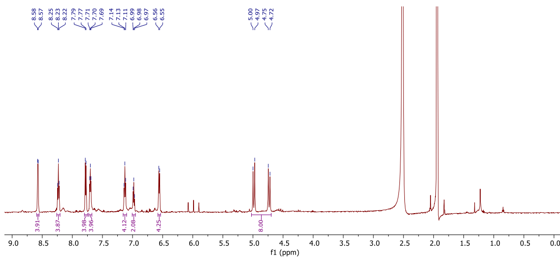
Slika D26. ^1\text{H} NMR spektar K2 , \text{CD}_3\text{CN} , 600 MHz, -40 °C.
