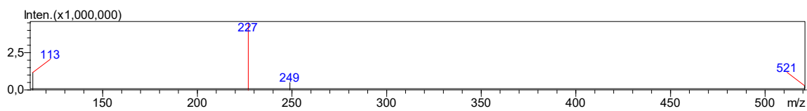
Slika D33. ESI-MS spektri L2. Pozitivan sken (gore) i negativan sken (dolje), metanol.
