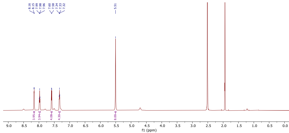
Slika D27. ^1\text{H} NMR spektar K4 , \text{CD}_3\text{CN} , 600 MHz, -40 °C.
