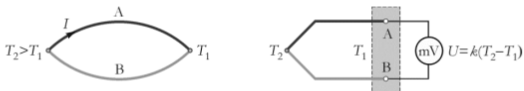
Slika 10 – Seebeckov efekt u termoparovima [10]
