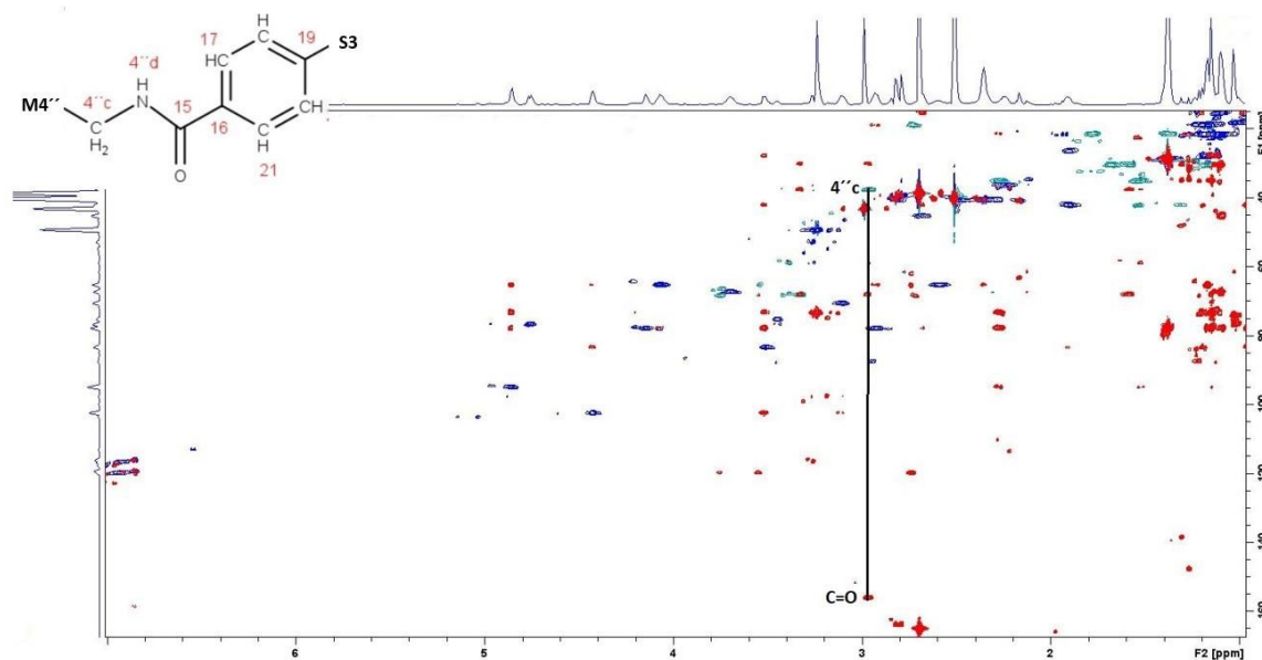
Slika 27. Uvećani dio preklapljenih spektara HSQC (plavo i zeleno) HMBC (crveno) spoja S4 i u rasponu od 0-8 ppm snimljen u DMSO- d_6 pri 298K s označenim korelacijskim signalima između protona H4''c i karbnilne skupine (C=O).
