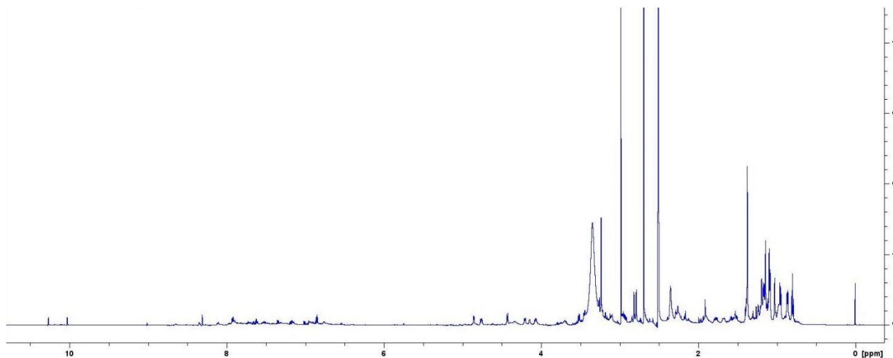
Slika 22. Spektar ^1\text{H} NMR spoja S4 snimljen u DMSO- \text{d}_6 pri 298 K.
