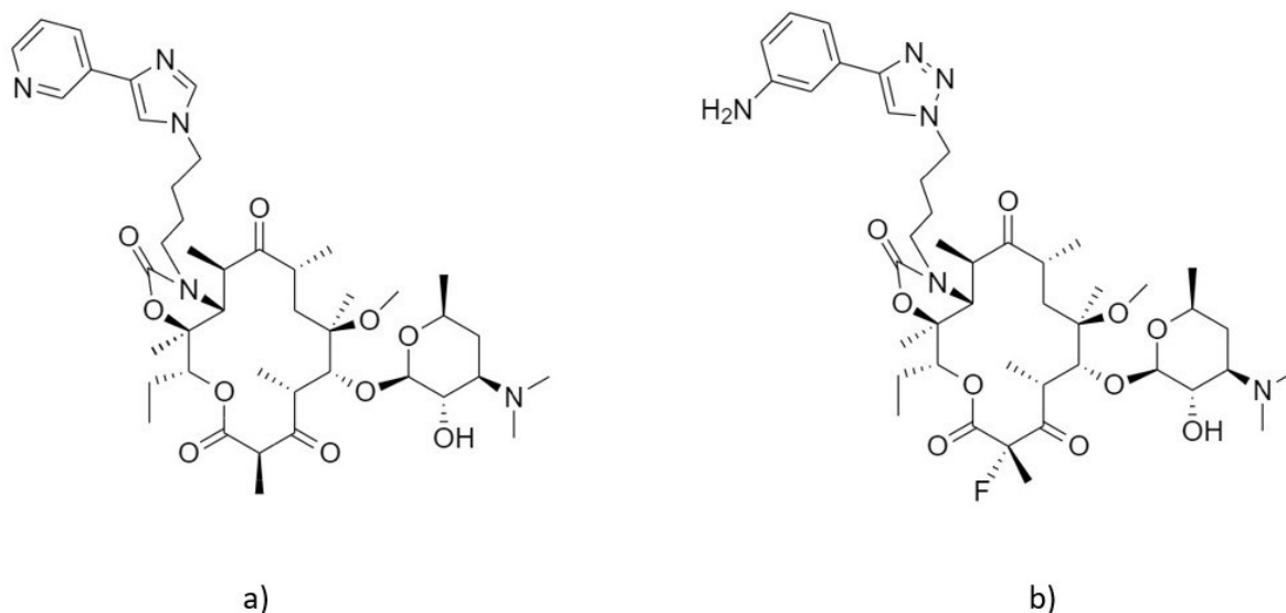
Slika 5. Strukturne formule predstavnika ketolida; a)telitromicin, b)solitromicin.
