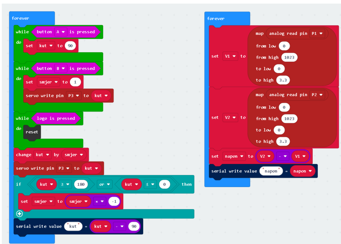
Slika 4.3: Programski kôd za mjerenje induciranog napona
