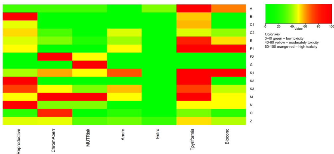
Slika 4.2. Toplinska karta parametara toksičnosti za 163 napuštena herbicida s prikazom udjela predviđenih toksičnih spojeva unutar svake pojedine HRAC klase herbicida. Herbicidi su grupirani u klase (Y-os) prema mehanizmu djelovanja na korov, a na X-osi su predviđene toksičnosti kod ljudi: reproduktivna/razvojna toksičnost ( Reproductive ), kromosomske aberacije ( Chrom_Aber ), mutagenost ( Ames test ) ( MUT_Risk ), afinitet za vezanje na androgenski receptor štakora ( Andro ), afinitet za vezanje na estrogenski receptor štakora ( Estro ), neurotoksičnost ( Tetrahymana pyrifomis inhibicija rasta Tpyrifomis ) i biokonzentracijski faktor ( Bioconc ). Legenda prikazuje stupanj toksičnosti od slabe do visoke toksičnosti prezentiran kroz spektar boja (zeleno – žuta – crveno).
