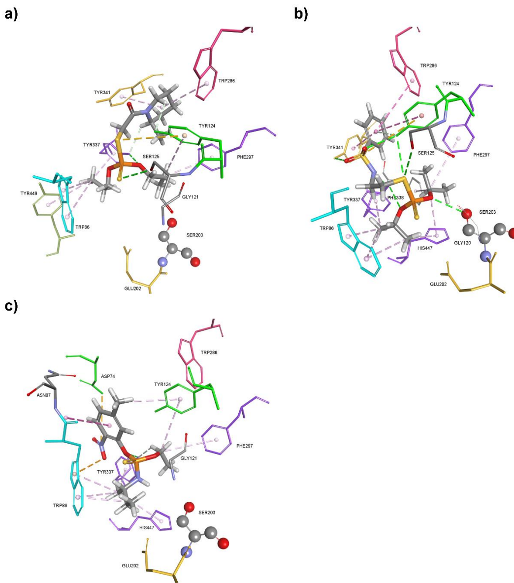
Slika 4.13. Model Michaelis-Mentena kompleksa herbicida: piperofos (a), benzulid (b) i butamifos (c) umutar aktivnog mjesta ljudske AChE (PDB: 4PQE) (prema Dym i sur. 143 ). Položaji su odabrani na osnovu kriterija gdje je odlazna skupina herbicida orijentirana nasuprot kisika (O) katalitičkog serina (Ser 203). Interakcije su prikazane isprekidanim linijama: hidrofobne (ružičasta), vodikove veze (zeleno) i elektrostatske (narančasta).
